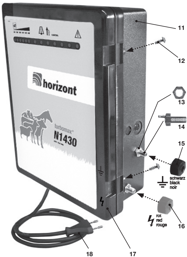
Fig. 2 Ersatzteile | Spare parts | Pièces détachées | Peças | Pezzi di ricambio | Reservecele | Reserve onderdelen | Części zapasowe | Запасные части
