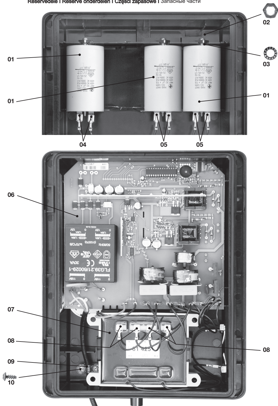
Fig. 1 Ersatzteile | Spare parts | Pièces détachées | Peças | Pezzi di ricambio | Reservedele | Reserve onderdelen | Części zapasowe | Запасные части
